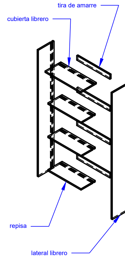
EXPLOSIVO
