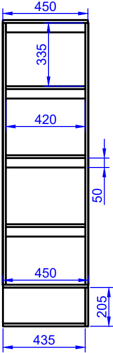
VISTA LATERAL
